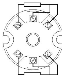
2xPT100 3+3 fili
