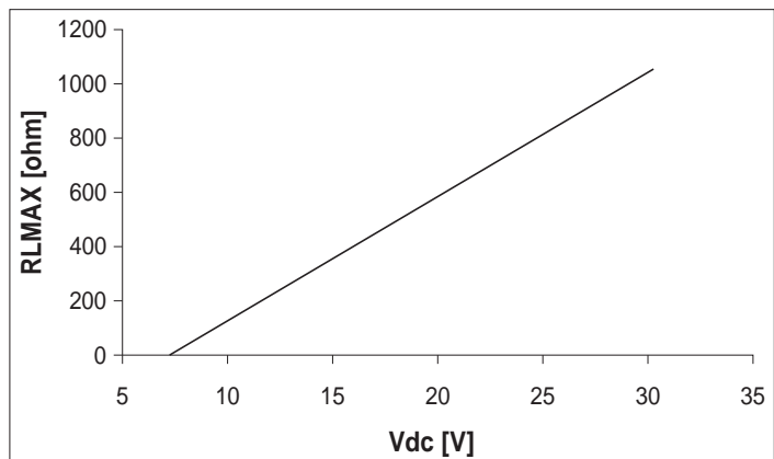
Fig. 3 Resistenza di carico in funzione della tensione di alimentazione.
