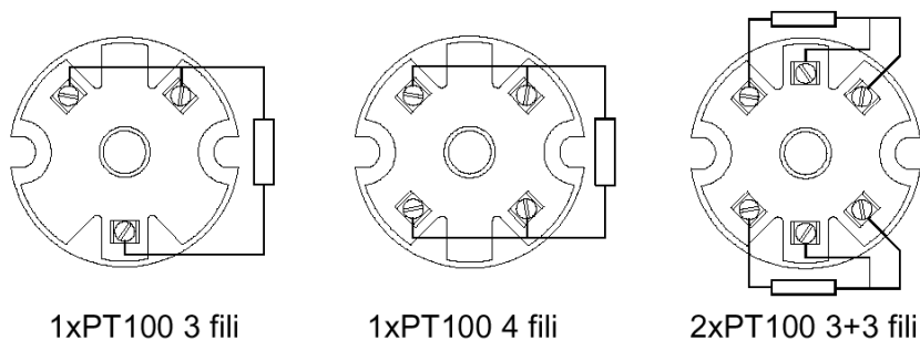
Schema di Collegamento Morsetti
