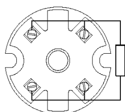
1xPT100 4 fili
