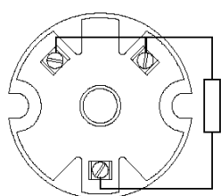
1xPT100 3 fili
