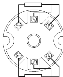
2xPT100 3+3 fili
